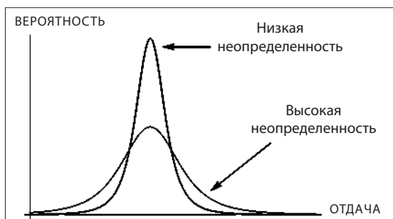
Рис. 25. Случай 1, симметрия. Когда система становится более непредсказуемой, мы переходим от одной «колокольной» кривой — первой, с узкой областью возможной отдачи, — ко второй, менее высокой, однако более растянутой. Соответственно увеличивается и вероятность положительных и отрицательных неожиданностей, то есть как позитивных, так и негативных Черных лебедей.
