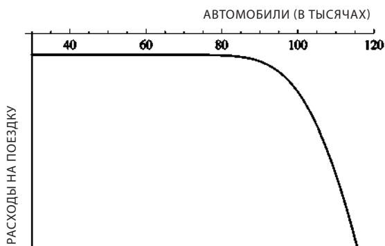
Рис. 14. График демонстрирует, что время поездки автора в аэропорт Кеннеди (и расходы на нее) после определенной точки нелинейно связаны с количеством машин на шоссе. Расходы на поездку обозначены кривой, которая изгибается внутрь, то есть вогнута, — а это нехорошо.
