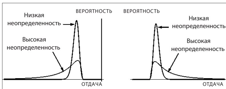
Рис. 26. Случай 2 (слева), хрупкость . Ограниченные приобретения, огромные потери. После увеличения уровня неопределенности в системе увеличивается вероятность в основном (иногда — только) отрицательной отдачи, строго негативного Черного лебедя. Случай 3 (справа), антихрупкость . Когда система становится хаотичнее и неопределеннее, повышается вероятность очень благоприятного исхода — и соответственно увеличивается ожидаемая отдача. С математической точки зрения это открытие эквивалентно анти-задержке самолета.
