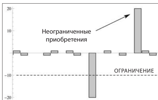
Рис. 24. Штанга во временном ряду. Ограничение отрицательной отдачи при сохранении положительной.
