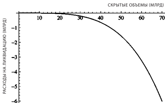
Рис. 15. Маленькое может быть красивым; оно точно менее хрупко. Затраты по сделке на графике — это функция от масштаба ошибки: они возрастают нелинейно, и мы видим, как они становятся мегахрупкими.
