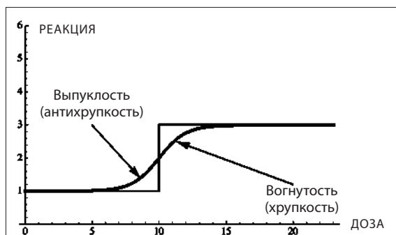
Рис. 32. Нелинейность в биологии. Выпукло-вогнутая кривая всегда наблюдается там, где некая переменная возрастает (монотонно, то есть никогда не убывает) и ограничена при этом минимальным и максимальным
