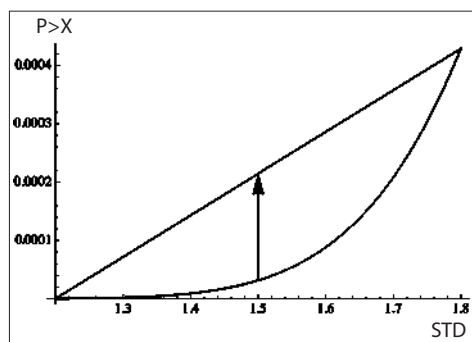
Рис. 38. В гауссовой модели вероятность выпукла в отношении среднеквадратического отклонения. График показывает, как среднеквадратическое отклонение (STD) влияет на вероятность P > x и сравнивает две ситуации: P > 6 при STD, равном 1,5, и P > 6 при линейной взаимосвязи в промежутке между 1,2 и 1,8 (здесь a(1) = 1/5 ).
