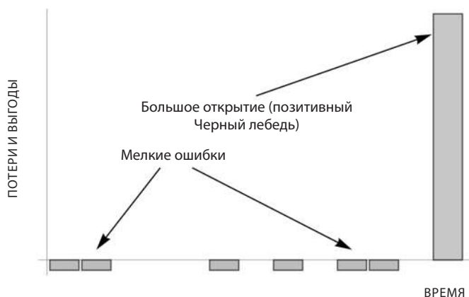
Рис. 6. Механизм «опциональных» проб и ошибок (модель «ошибайся часто»), или выпуклое прилаживание. Малозатратным ошибкам, максимальный убыток от которых известен, сопутствует большая (неограниченная) потенциальная прибыль. Это основное свойство позитивных Черных лебедей: выгоды от них ничем не ограничены (в отличие от лотерейных билетов) или, если точнее, предел таких выгод неизвестен; при этом урон от ошибок ограничен и известен.
