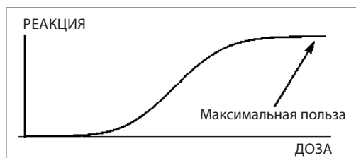
Рис. 29. Слабая антихрупкость (Среднестан) с ограниченным максимумом. Типична для природы.
