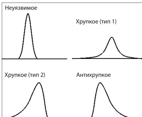
Рис. 22. На горизонтальной оси отображается отдача, на вертикальной — вероятность этой отдачи. Неуязвимое : малая положительная и отрицательная отдача. Хрупкое (тип 1) , очень редкий: отдача может быть как большой положительной, так и большой отрицательной. Почему это редкий тип? Подобная симметрия очень, очень, очень
