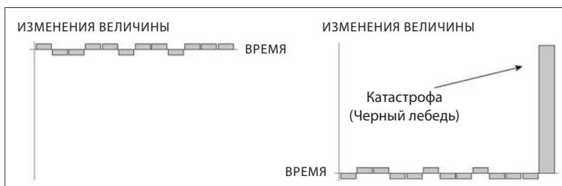
Рис. 21. Неуязвимое (но не антихрупкое) (слева): величина все время меняется незначительно или не меняется вообще. Значительных скачков не бывает. Антихрупкая система (справа): благодаря неопределенности мы приобретаем куда больше, чем теряем, — полная противоположность первому графику на рис. 20.
