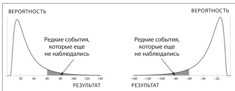
Рис. 35. Антихрупкость, обратная проблема индюшки: редкое, еще не наблюдавшееся событие — позитивное. Взглянув на позитивно скошенный (антихрупкий) временной ряд и сделав вывод о ненаблюдаемости события,
