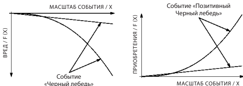
Рис. 13. Два примера уязвимости, один линейный, другой нелинейный: на графике слева — с негативной выпуклостью, иначе говоря, вогнутый; на графике справа — с позитивной выпуклостью. Непредвиденное событие воздействует на обладающий нелинейной уязвимостью объект все больше и больше. Чем масштабнее событие, тем больше разница.
