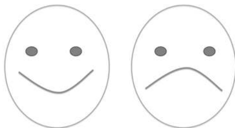
Рис. 11. Улыбайтесь! Лучший способ понять выпуклость и вогнутость. То, что искривлено в направлении вовне, выглядит как улыбка, а то, что внутрь, — кажется грустным лицом. Выпуклое (слева) антихрупко, вогнутое (справа) хрупко (страдает от эффекта негативной выпуклости).
