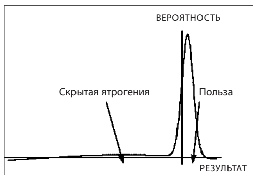
Рис. 31. Медицинская ятрогения: случай маленьких приобретений и огромных потерь а-ля Черный лебедь в пространстве вероятностей. Ятрогения имеет место, когда скромная очевидная польза (скажем, когда мы, приняв лекарство, избавляемся от небольшого дискомфорта или неопасной инфекции) сочетается
