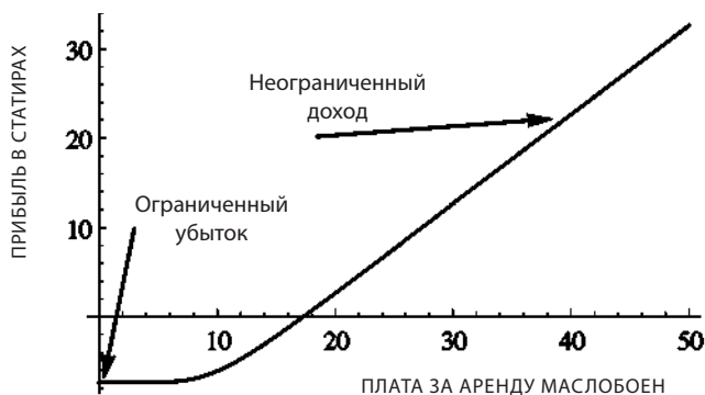
Рис. 5. Антихрупкость Фалеса. Он платит мало, а получить может много. Между выгодой и потерями наблюдается асимметрия.
